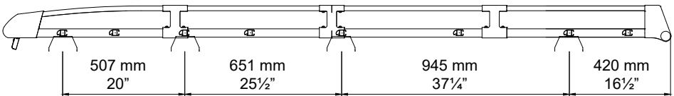
Vivaro (14→), Trafic (14→), Talento/NV300 (16→) L2H2
